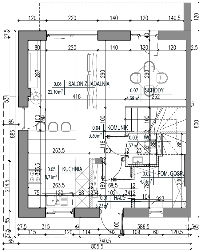
RZUT PARTERU
