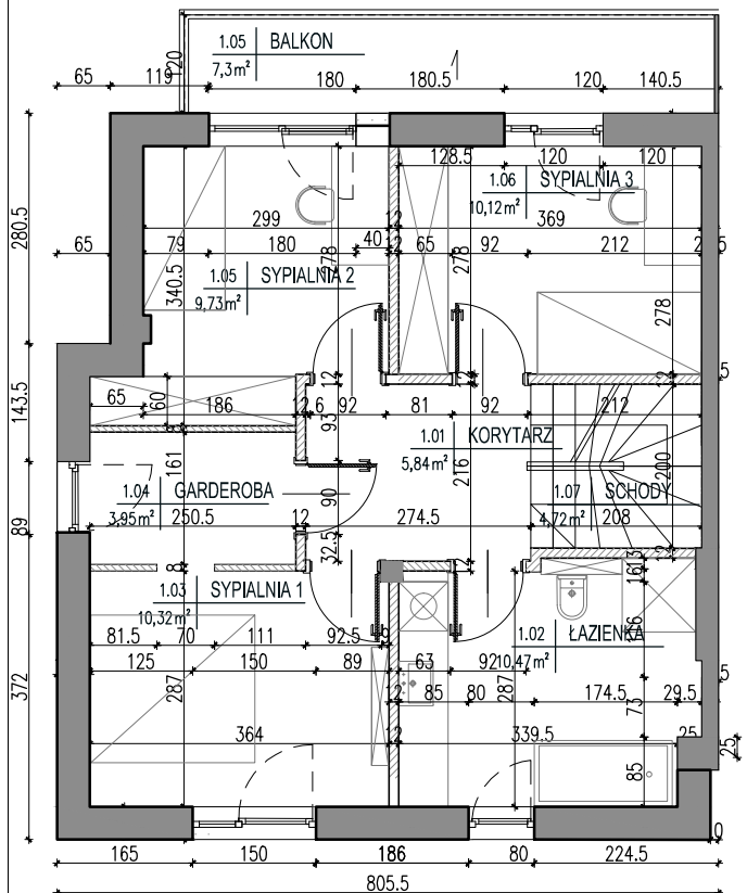
RZUT PIĘTRA
