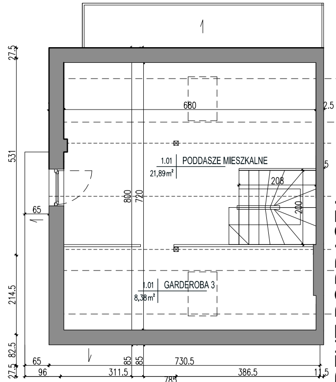
RZUT PODDASZA
