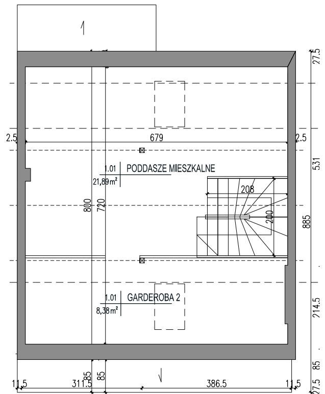
RZUT PODDASZA
