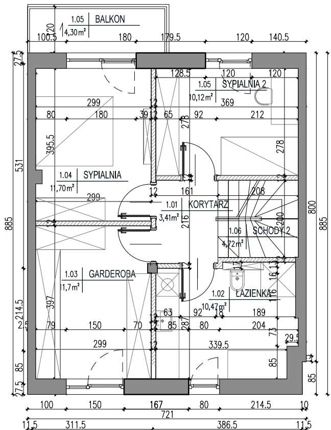
RZUT PIĘTRA
