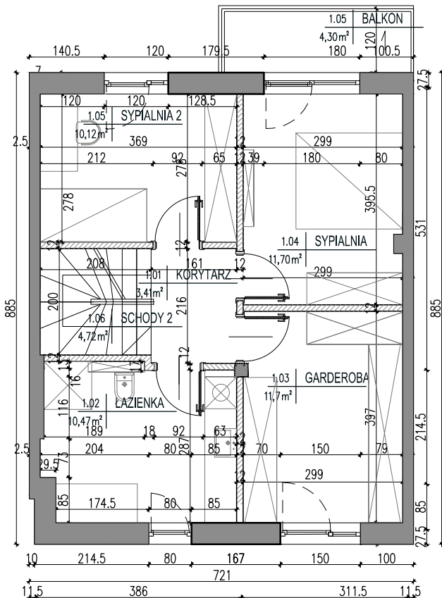
RZUT PIĘTRA
