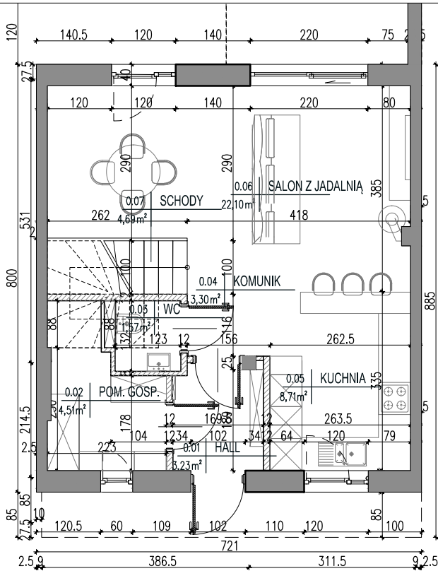
RZUT PARTERU
