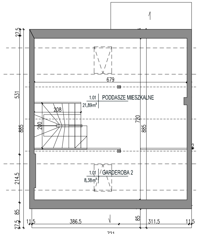
RZUT PIĘTRA
