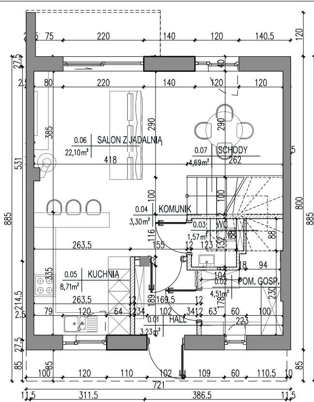
RZUT PARTERU
