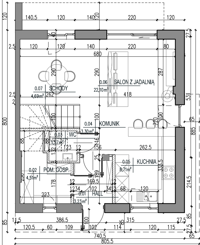
RZUT PARTERU
