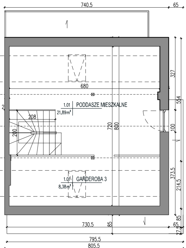
RZUT PIĘTRA
