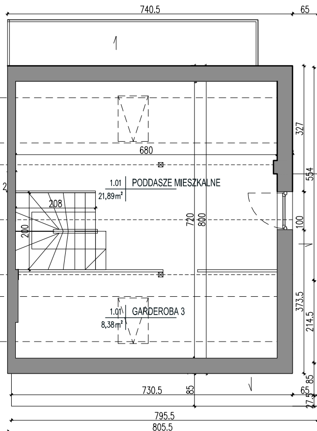
RZUT PIĘTRA
