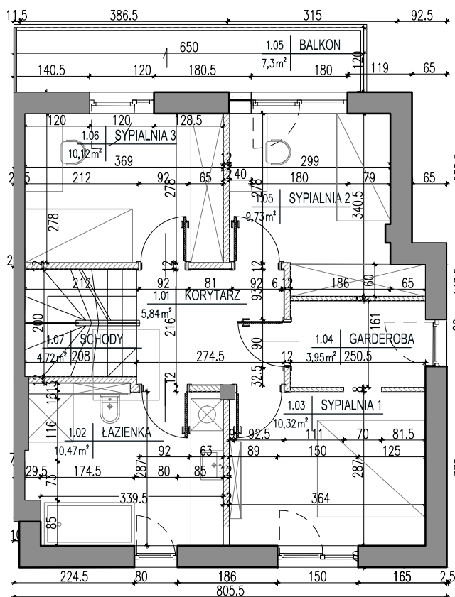
RZUT PIĘTRA
