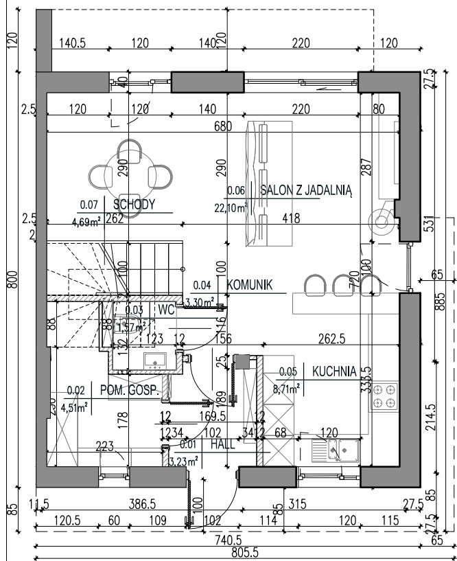
RZUT PARTERU
