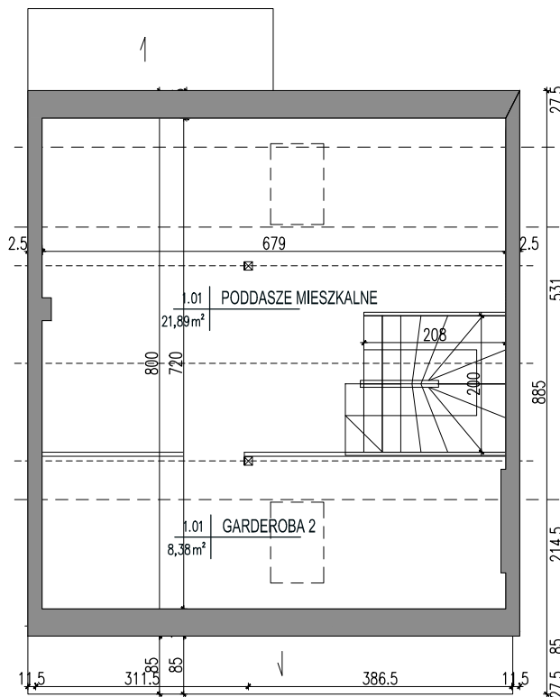
RZUT PODDASZA
