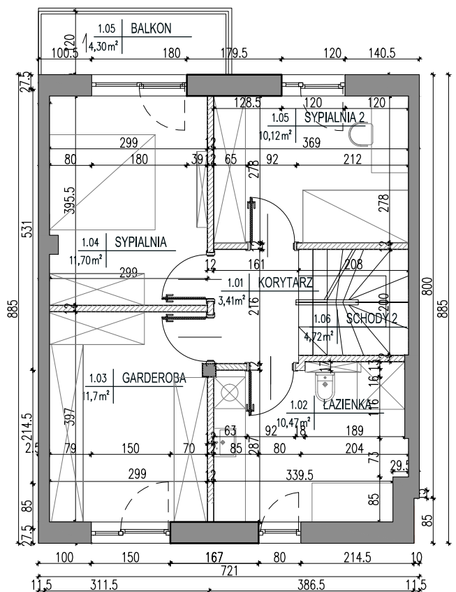
RZUT PIĘTRA
