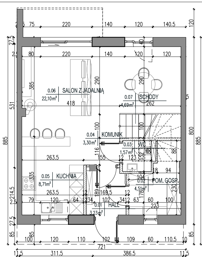
RZUT PARTERU
