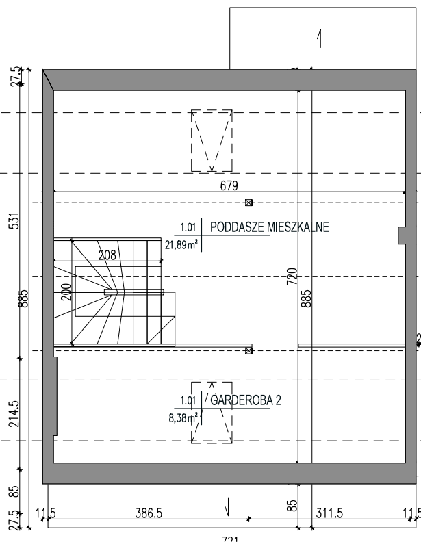
RZUT PODDASZA
