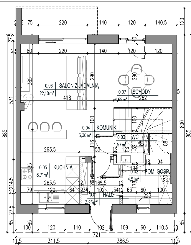
RZUT PARTERU
